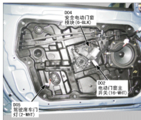
74. 驾驶席车门
