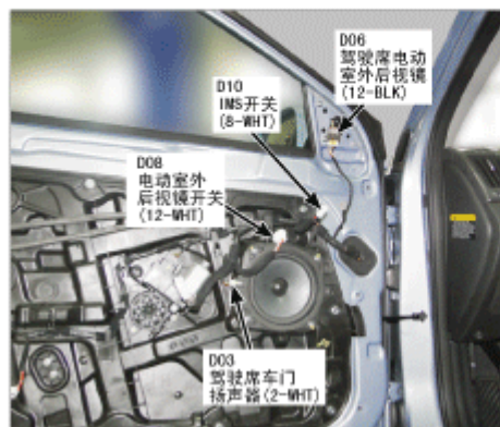
73. 驾驶席车门
